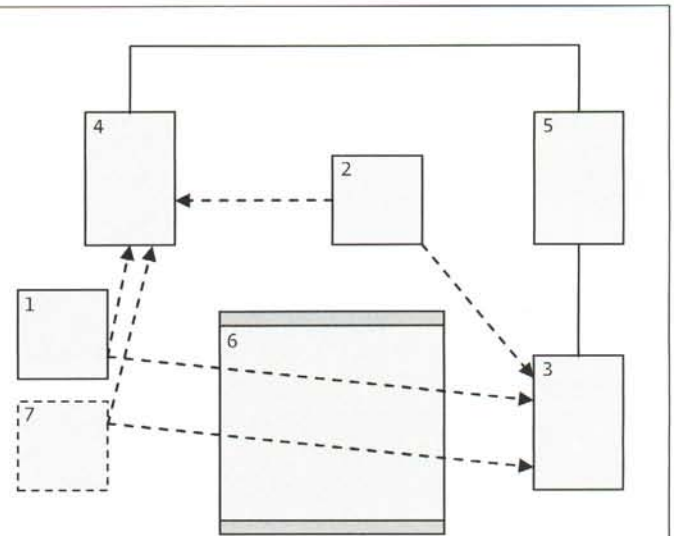
Рис.1. Блок-схема ГА с коррекцией сигналов фотоприемников: 1 – "измерительный" СД; 2 – "калибровочный" СД; 3 – "измерительный" фотоприемник; 4 – опорный фотоприемник; 5 – блок обработки сигналов; 6 – ячейка с анализируемым (поглощающим излучение) веществом; 7 – дополнительный светодиодный излучатель Fig. 1. Flow chart of GA with correction of photodetector signals: 1 – "measuring" LED; 2 – "calibrating" LED; 3 – "measuring" photodetector; 4 – bearing photodetector; 5 – unit for signal processing; 6 – cell with analyzed (radiation absorbing) material; 7 – additional light emitter
